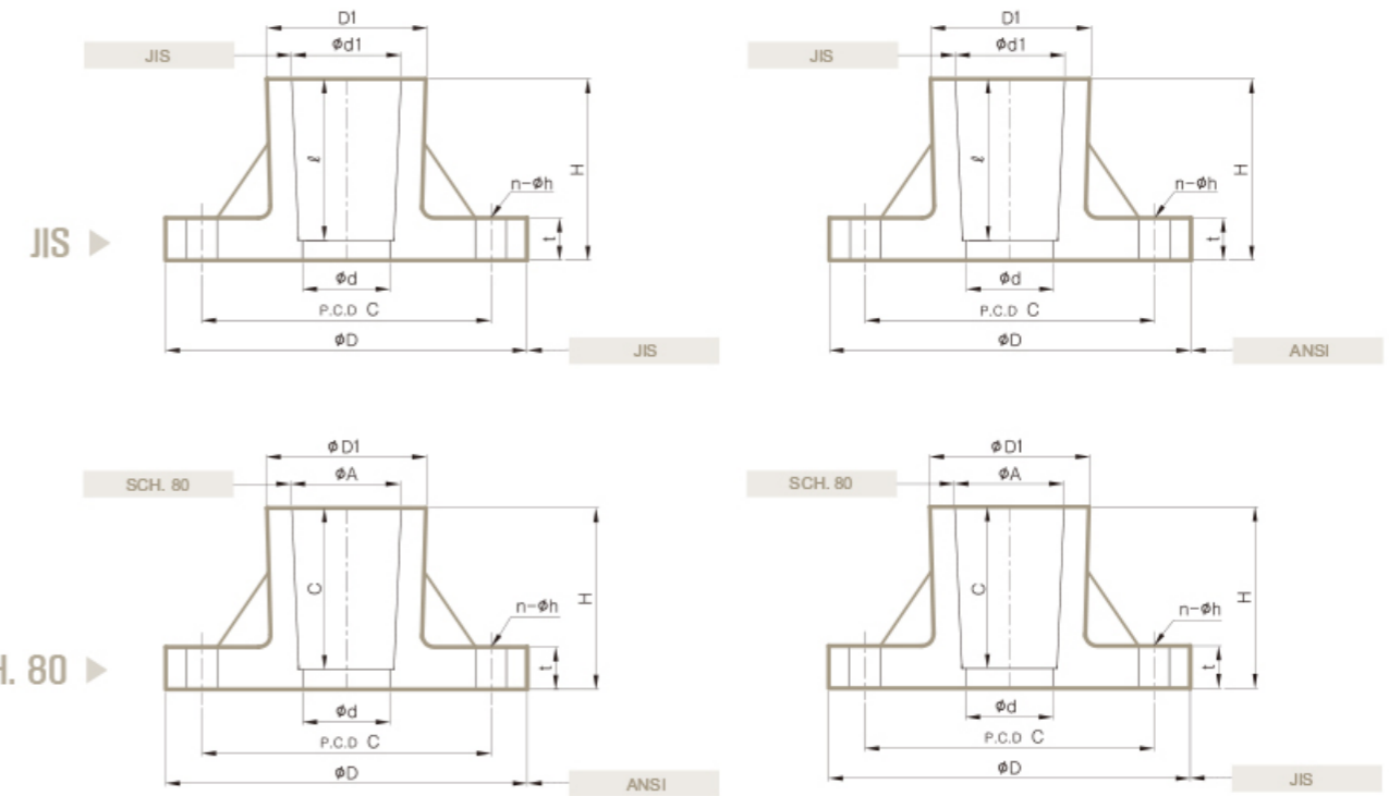
SCH. 80 + ANSI (SOCKET : SCH. 80 / FLANGE HALL : ANSI)
